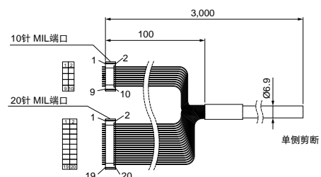
并行通信 / ON/OFF输入用分支线缆 EXCB2-M10M20-3(3m)
