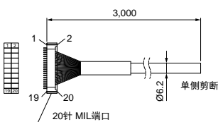
并行通信用线缆 EXCB2-M20-3(3m)
