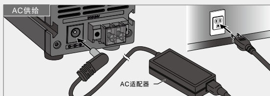
AC100-240V输入需使用AC适配器 (选件)。 型号: ADP2460-PFB-JTLV6 (遵从美国DoE CEC Level VI外置电源规定)
