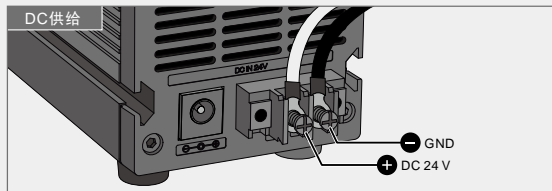
DC24V输入使用主体背面的端子排。
