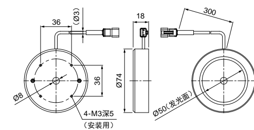
LKR-70-8SW2/BL2/GR2的发光面为Ø49.2
