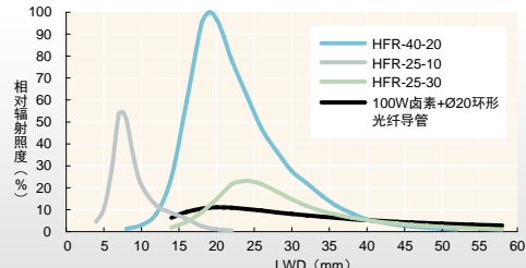
HFR 系列各 LWD 的辐射照度变化图表
